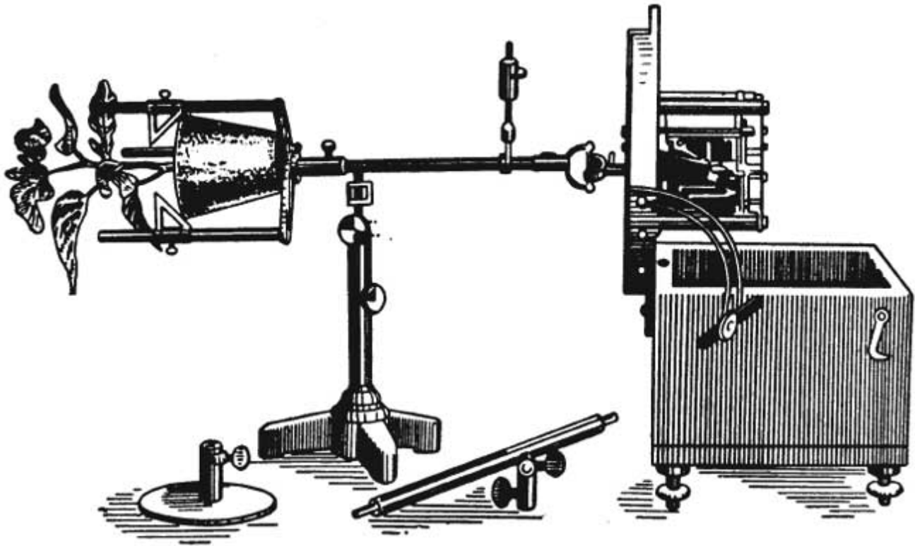
Клиостат, на котором работал В.В. Сапожников
